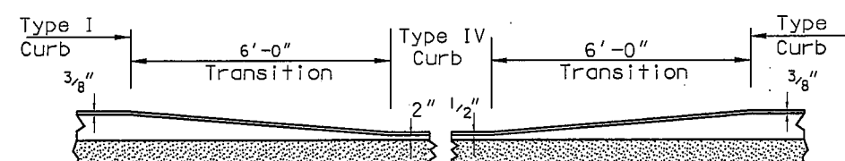
SECTION A-A
