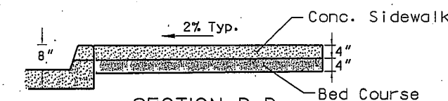
SECTION D-D
